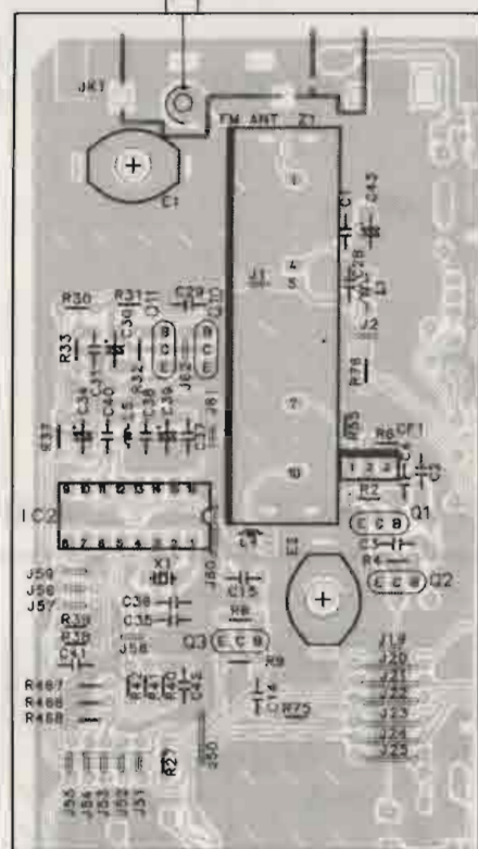
E MAIN/TUNER P.C.B. (REP1378A....E,EB) (REP1378B....EG) (REP1378E....GN)
