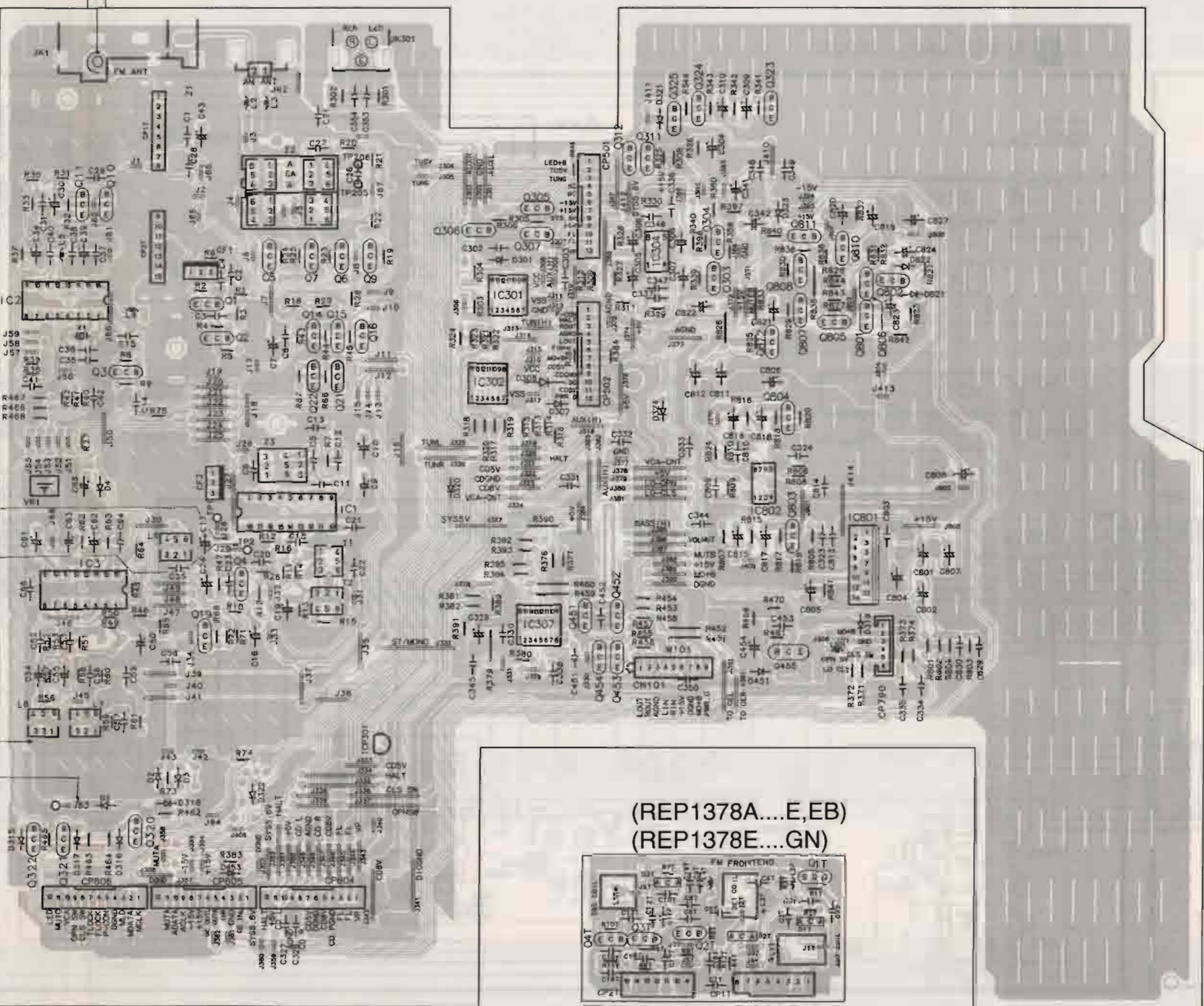
M TUNER BLOCK P.C.B.
