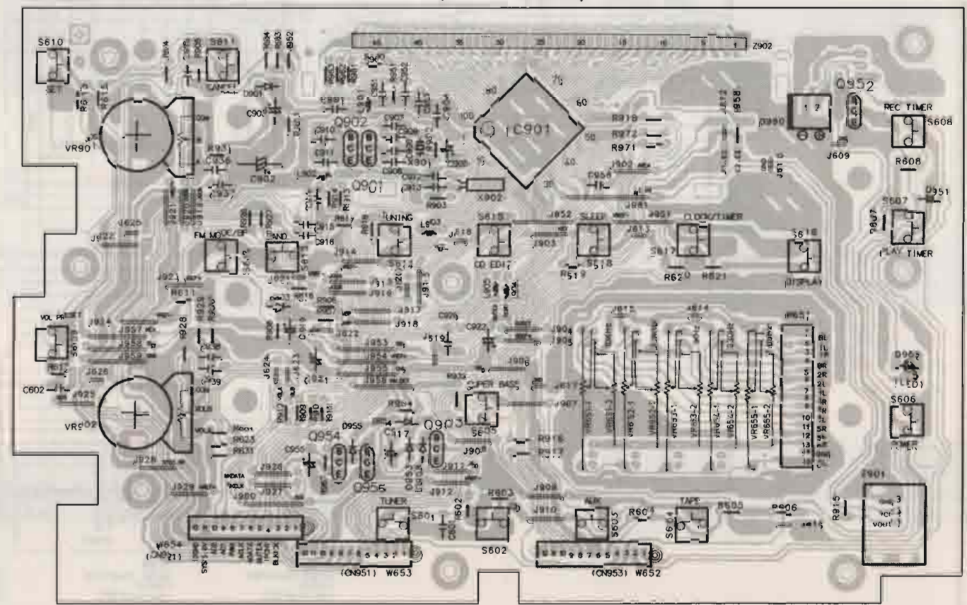
L PANEL P.C.B. (MICROCOMPUTER) (REP1381A)
